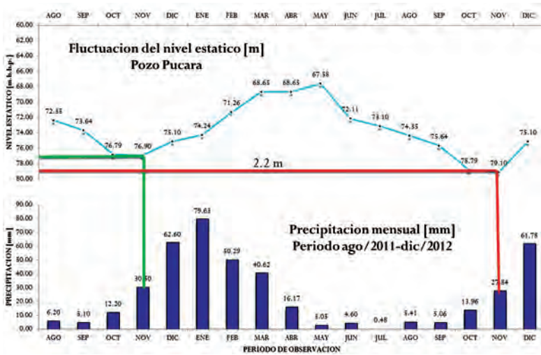
Figura 4.8. Variación anual en el nivel piezométrico del Pozo Pucara
